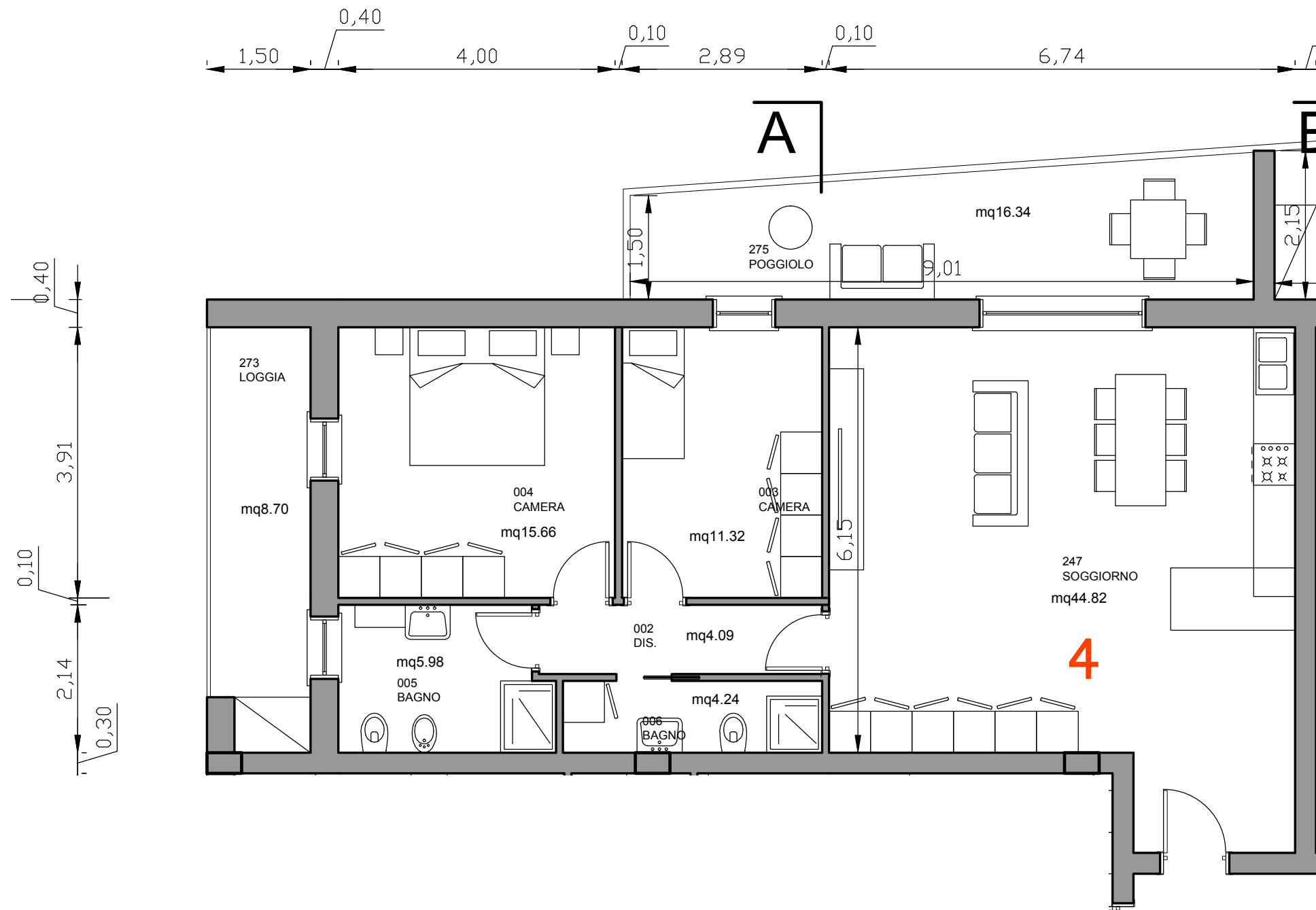
UNITÀ 4 - PLANIMETRIA - PRIMO PIANO
