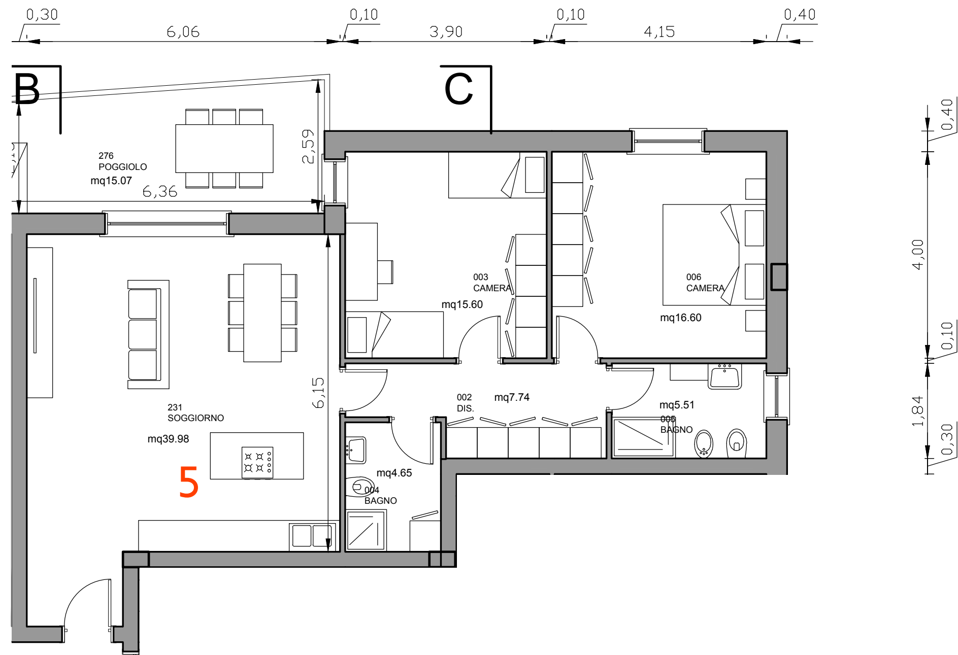
UNITÀ 5 - PLANIMETRIA - PRIMO PIANO
