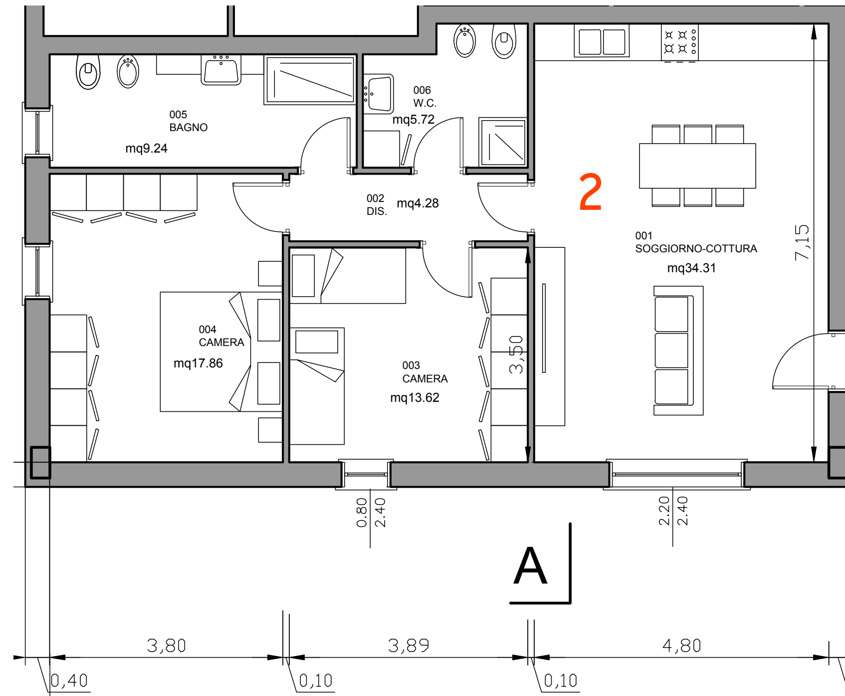
UNITÀ 2 - PLANIMETRIA - PIANO TERRA
