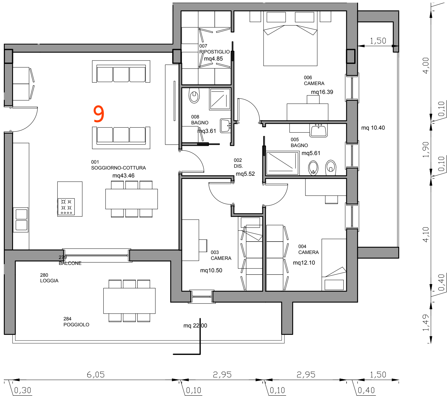
UNITÀ 9 - PLANIMETRIA - SECONDO PIANO
