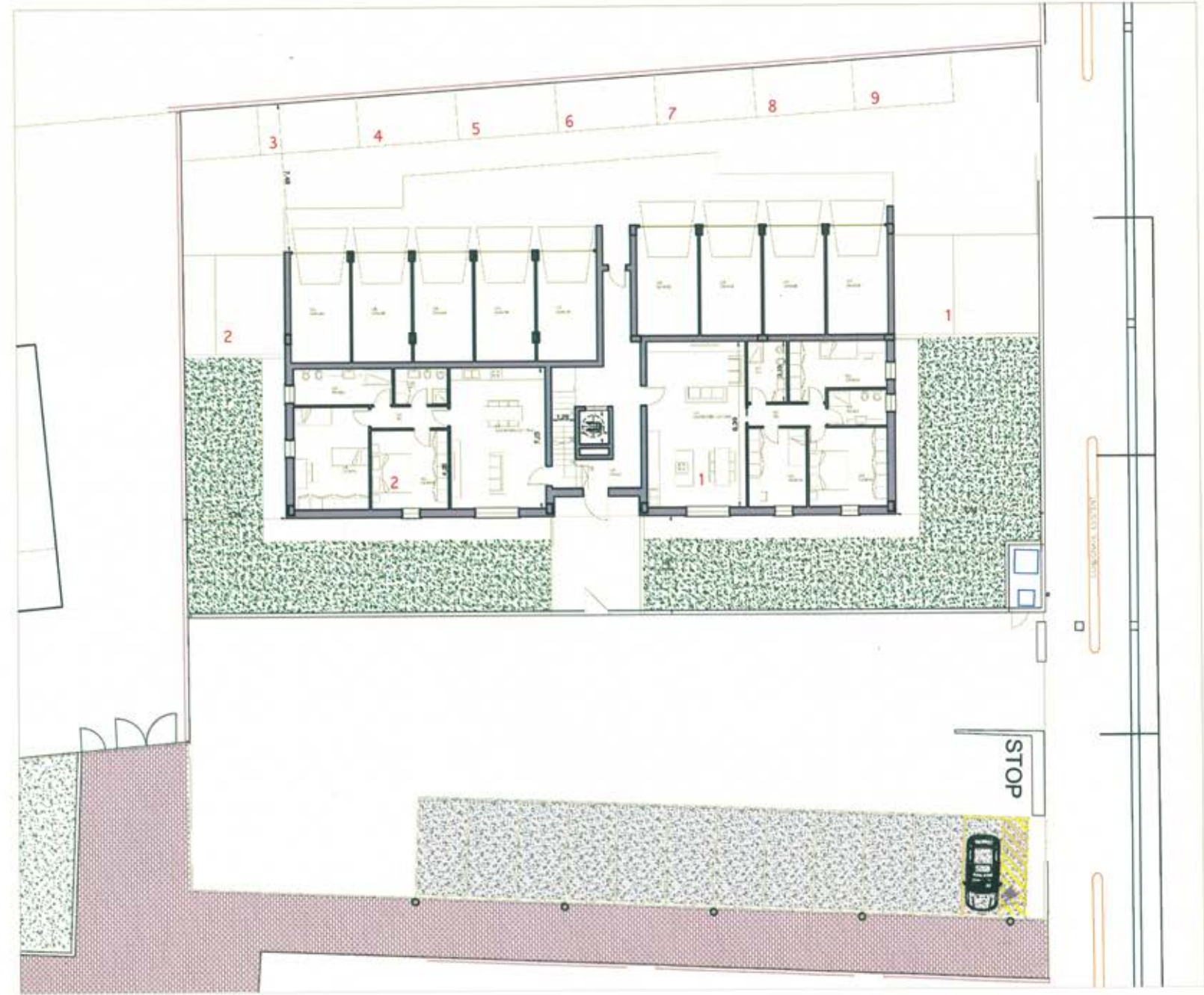
PLANIMETRIA GENERALE SPAZI ESTERNI
