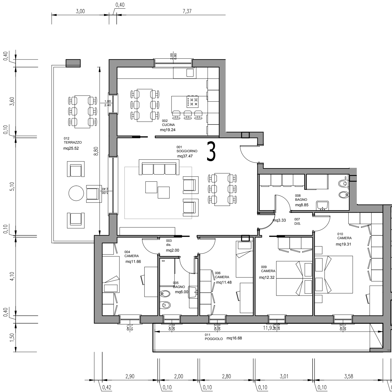
UNITÀ 3 - PLANIMETRIA - PRIMO PIANO
